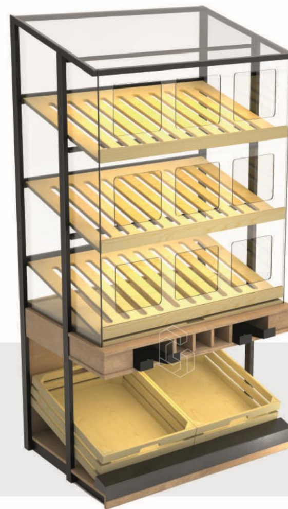
Хлебный стеллаж №4 С отверстиями 3 полки ш1000 гл700 в1950
