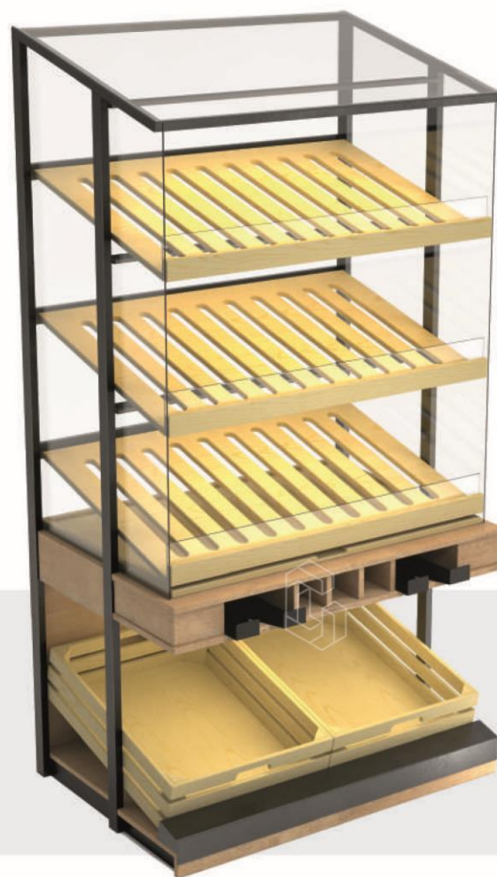
Хлебный стеллаж №4 Открытый 3 полки ш1000 гл700 в1950
