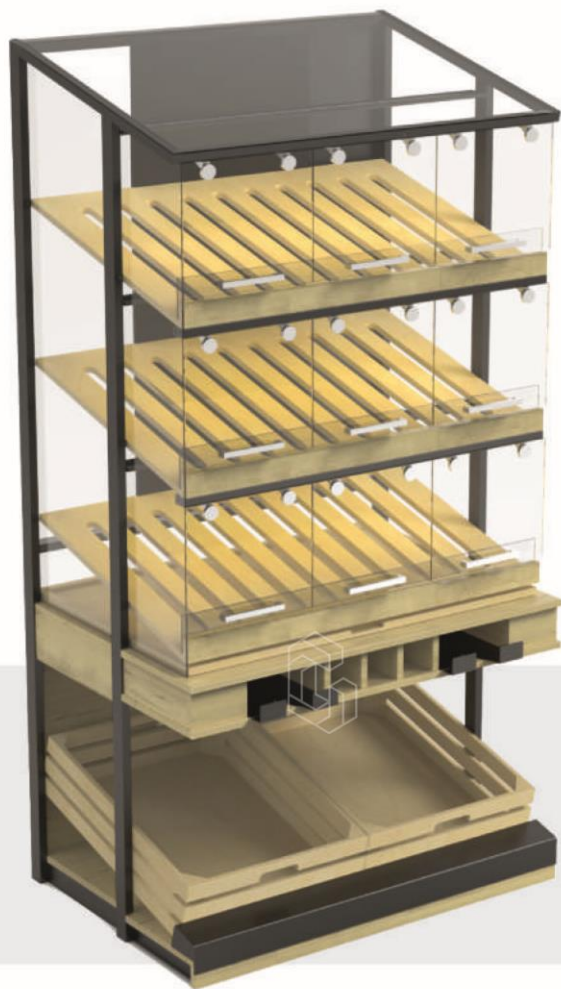
Хлебный стеллаж №4 Закрытый 3 полки 9 дверок ш1000 гл700 в1950
